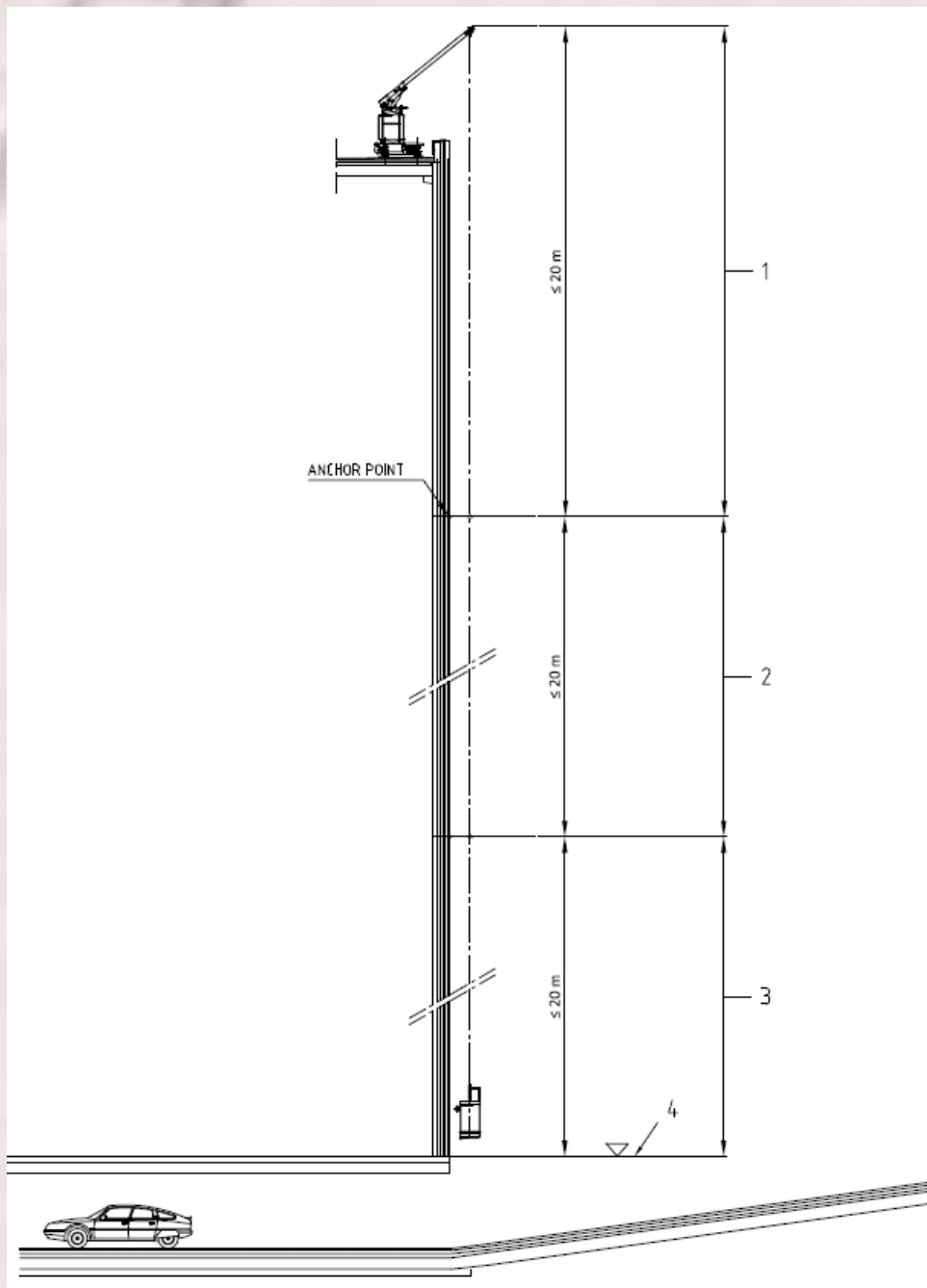
Figuur GG-03 Gevelonderhoudsinstallatie met op meerdere niveaus gevelpunten
