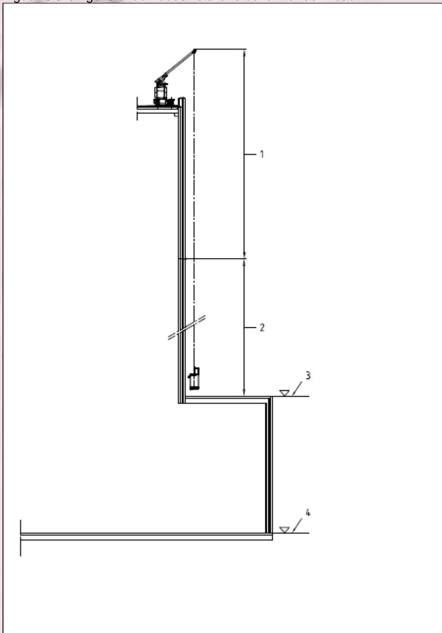
Figuur GG-04 gevelonderhoudsinstallatie boven terrasniveau
